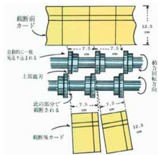
（ロータリー裁断解説図）
